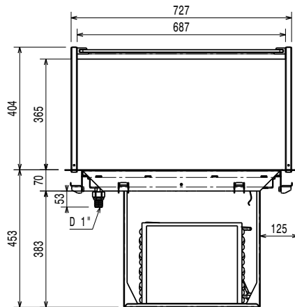
Front aanzicht
