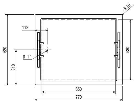
Boven aanzicht
